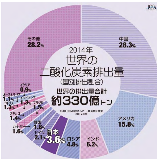
図 1-1-5 世界全体の二酸化炭素排出量 (平成26年 (2014年))
