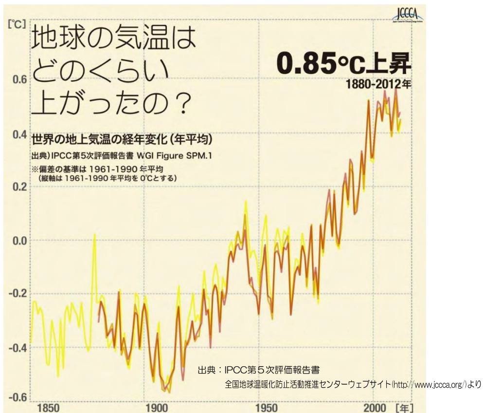
図 1-1-2 地上の平均気温の増減
