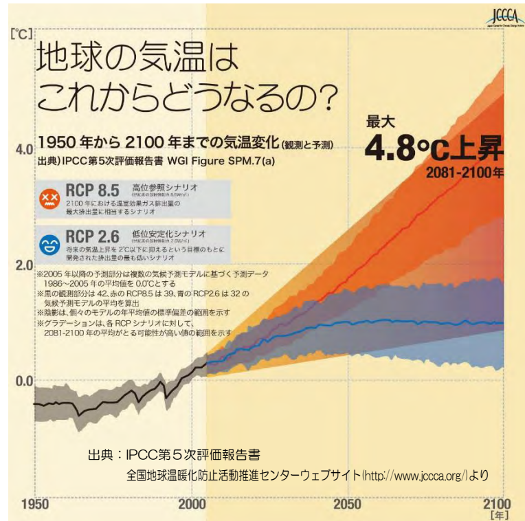
図 1-1-3 2100年までの気温変化の予測
