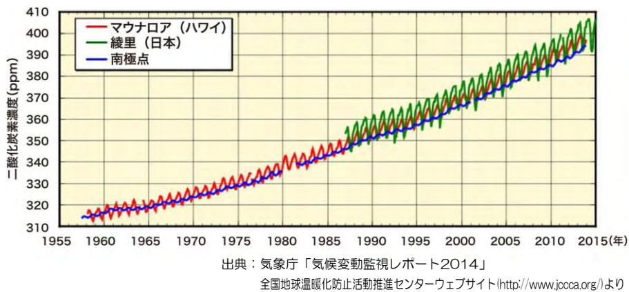
図 1-1-1 二酸化炭素濃度の経年変化
