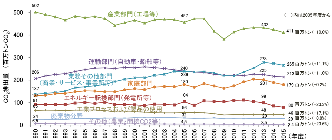
図 1-1-7 日本の部門別二酸化炭素排出量の推移
