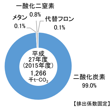
図 1-1-29 平成27年度（2015年度）のガス別排出量
