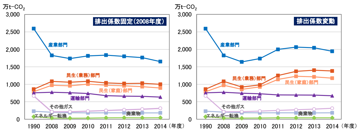
図 1-1-8 大阪府域の温室効果ガス排出量の推移
